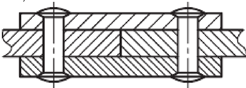
Рис. 18. Штриховка смежных сечений
